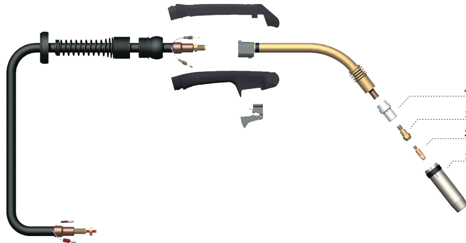
1. Газовое сопло (L=84)
